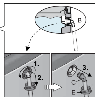
En option : démonter la pièce de raccordement du trop-plein de sécurité
