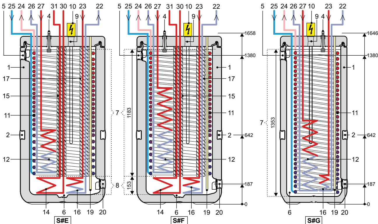
Fig. 3-2 Raccordements et dimensions, Ballon d'eau chaude haute performance avec appoint solaire - types HYC-P
