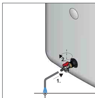
Fig. 6-1 Processus de vidange sans p=0 système solaire
