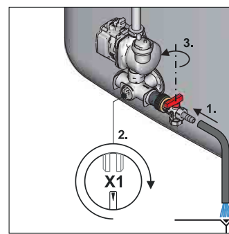
Fig. 6-2 Processus de vidange avec p=0 système solaire
