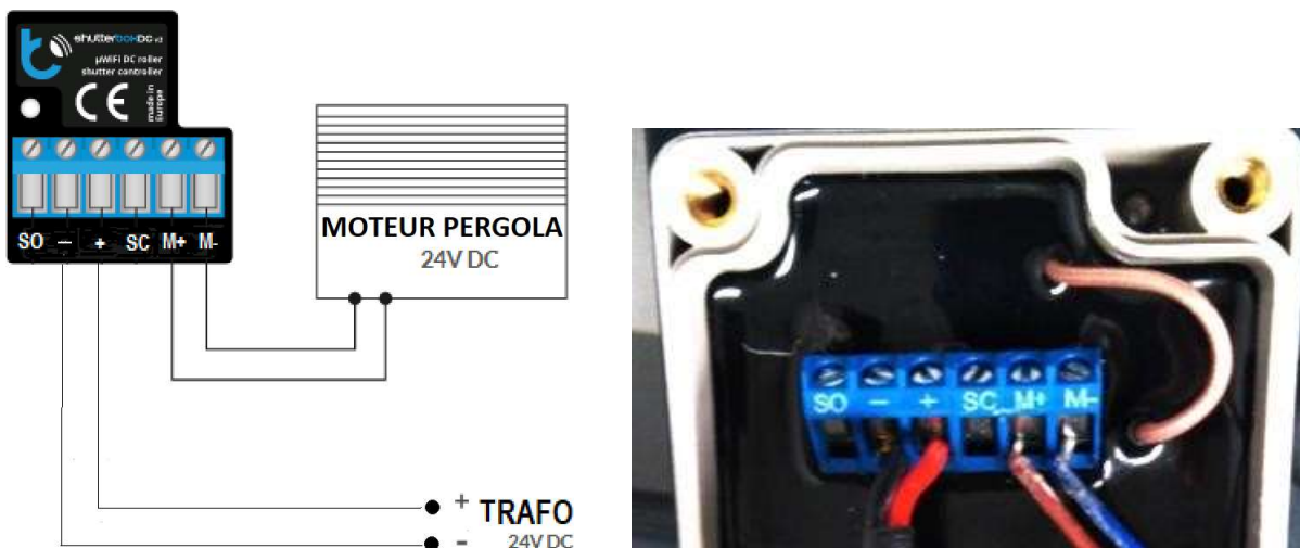
Fig. 36 Schéma de câblage de l'unité de commande Pergola DC (fabriquée en usine)
