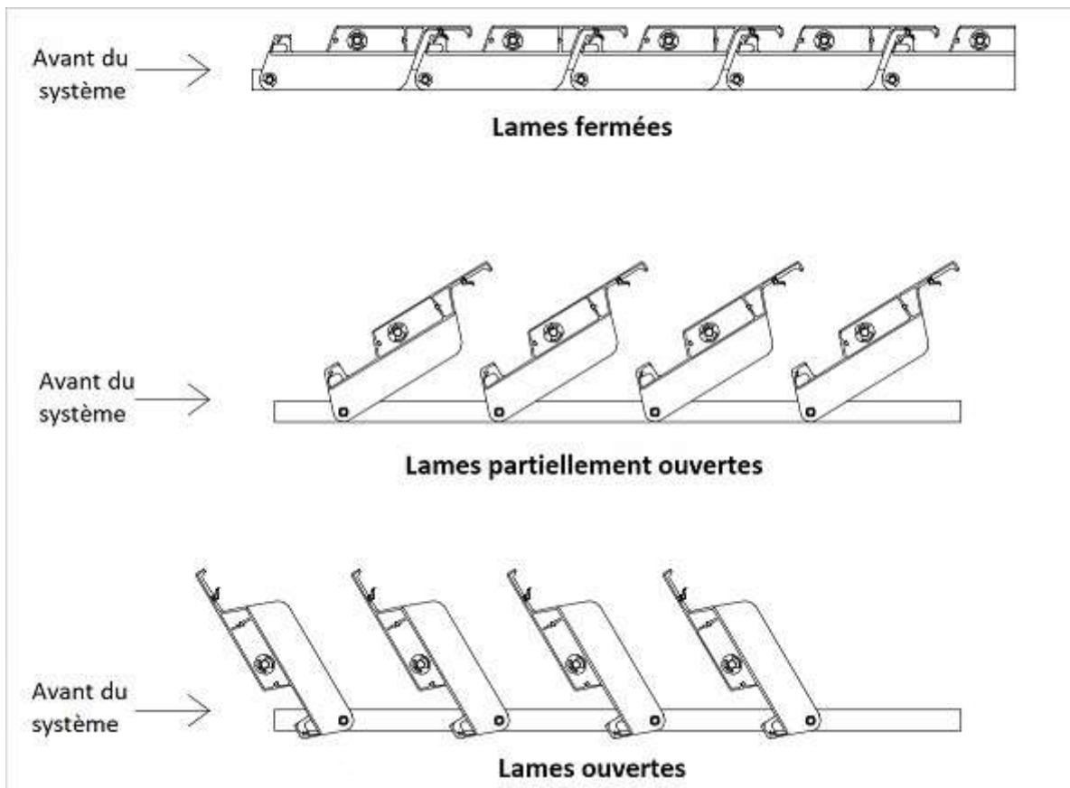
Fig. 2. Réglage standard du sens d'ouverture des lames pour la Pergola STANDARD
