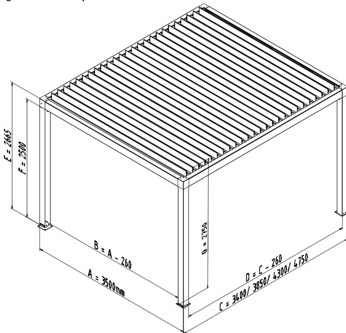
Fig. 1. Pergola Standard autoportante
