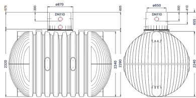
Mesure - [mm]
