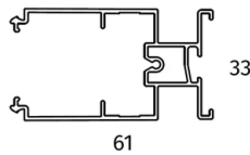
Barre de charge 33x61mm
