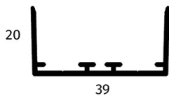
Profil mural 39x20mm
