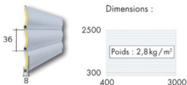
Tablier ALU DP 368
